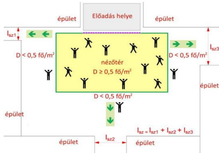
7. ábra: A kezdeti szabad menekülési szélesség zöld vonallal, a menekülésre figyelembe vett útvonalak legkisebb szabad szélességeinek összege piros méretezővel szemléltetve (a második számítási módszerhez kapcsolódó ábra)
